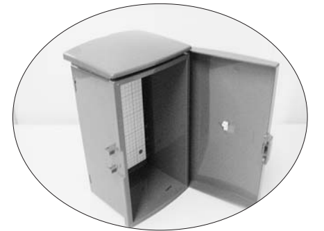
放送用光受信機収納箱 縦約35cm、横約20cm、奥行き約15cm
